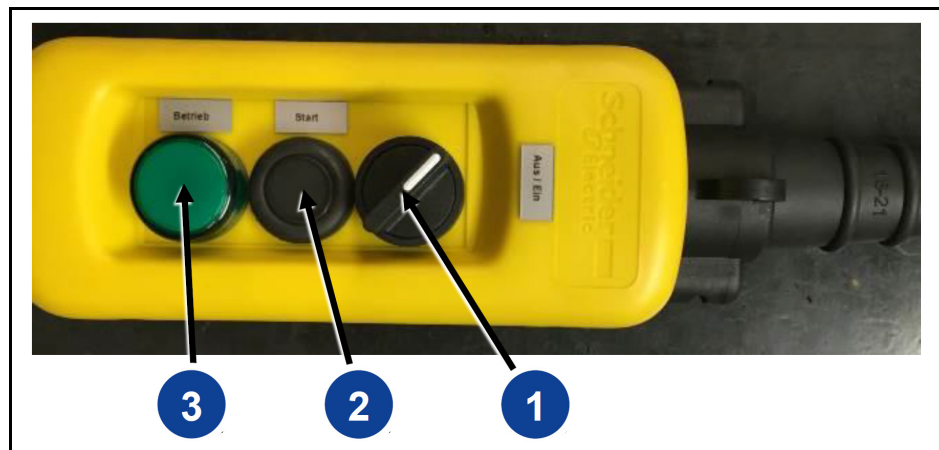
Abb. 8-4 Kabel-Fernbedienung
