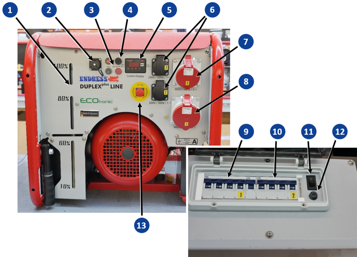
Abb. 6-4 Komponenten des Bedienfelds full option
