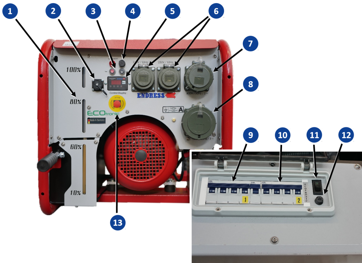
Abb. 6-5 Komponenten des Bedienfelds SEA
