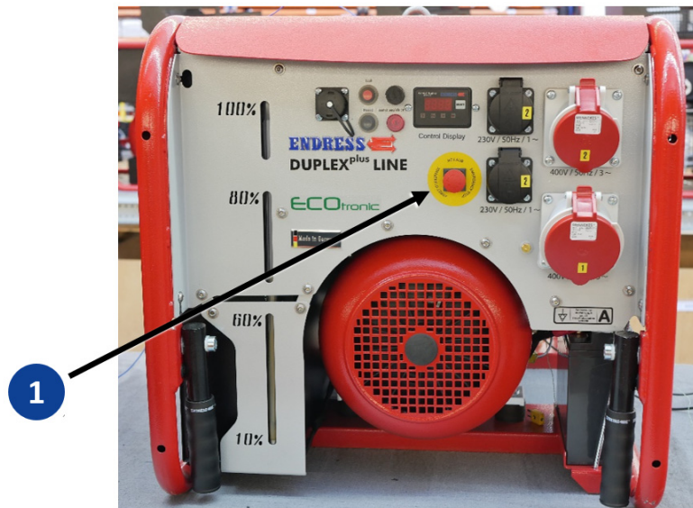
Abb. 7-3 NOT-AUS-Schalter
